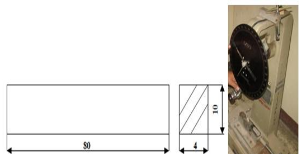
Gambar 1. Dimensi spesimen impak (satuan dalam milimeter) dan alat uji
