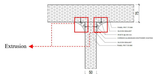
(b) Detail Sambungan Partisi dan Plafon
