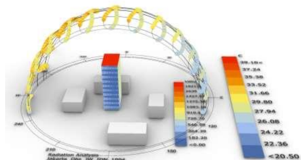
Gambar 3. Simulasi Radiasi dan Pergerakan Matahari dengan Desain Fasad Usulan Sumber : Peneliti (2019)
